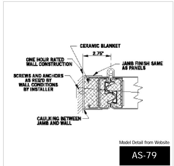
Hinged Jamb
