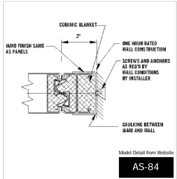
Variable Fixed Jamb
