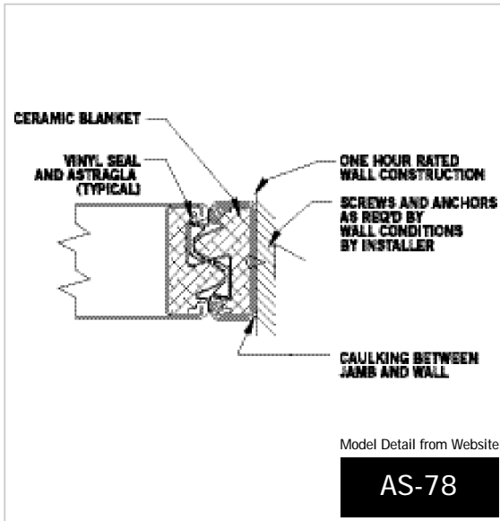
Nominal Fixed Jamb
